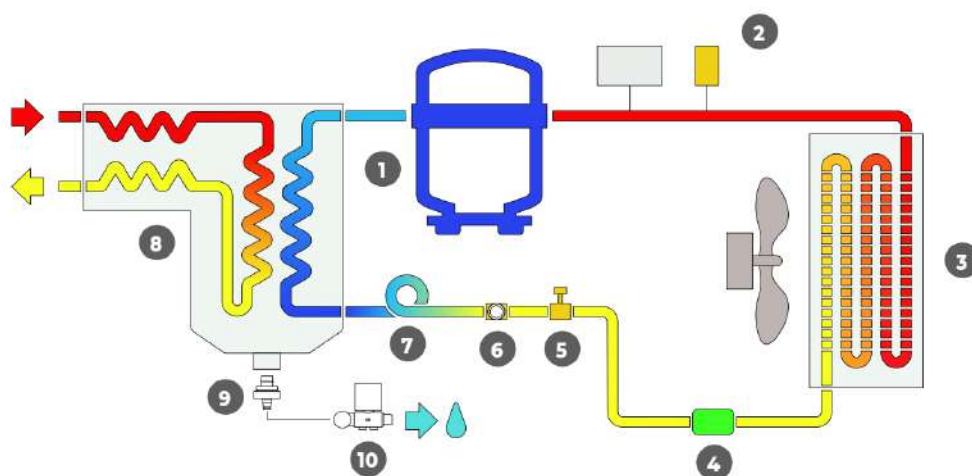
Schéma de principe d'un sécheur air comprimé à détente directe
