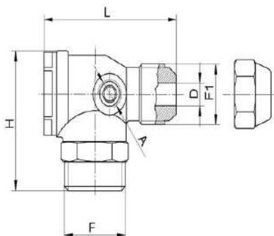
Raccordement M-M
