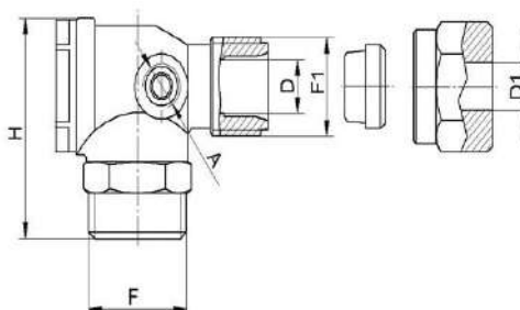
Raccordement M-Olive
