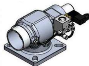
CLAPET C90E
